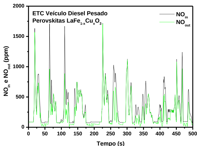
FIGURA 2. Simulação do ciclo de condução ETC Veículo Diesel Pesado quando este é equipado com o catalisador SCR LaFe 1-x Cu x O 3 .
