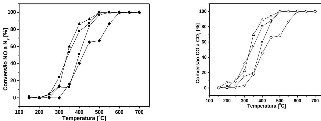
FIGURA 4. Conversão de CO a CO 2 sobre as perovskitas: (◇) LaFeO 3 ; (○) LaFe 0.8 Cu 0.2 O 3 ; (△) LaFe 0.5 Cu 0.5 O 3 ; (□) La 2 CuO 4 .
