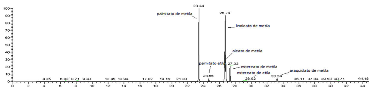
Figura 4. Cromatograma do possível biodiesel obtido com óleo da borra de café.
