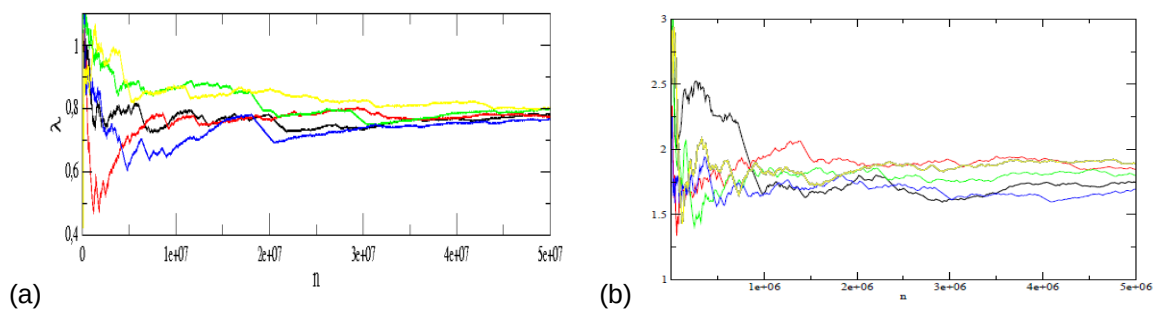
Figura 3: Convergência dos Expoentes de Lyapunov para os Modelos Completo (a) e Simplificado (b) do Acelerador de Fermi.
