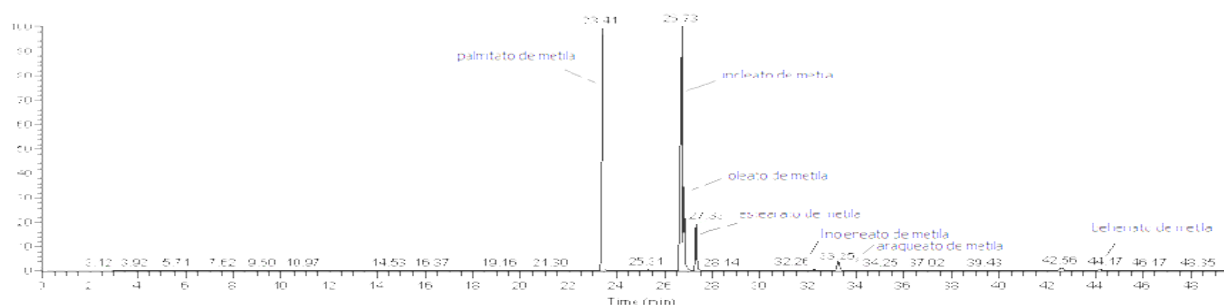
Figura 4. Cromatograma do possível biodiesel obtido com óleo da borra de café.
