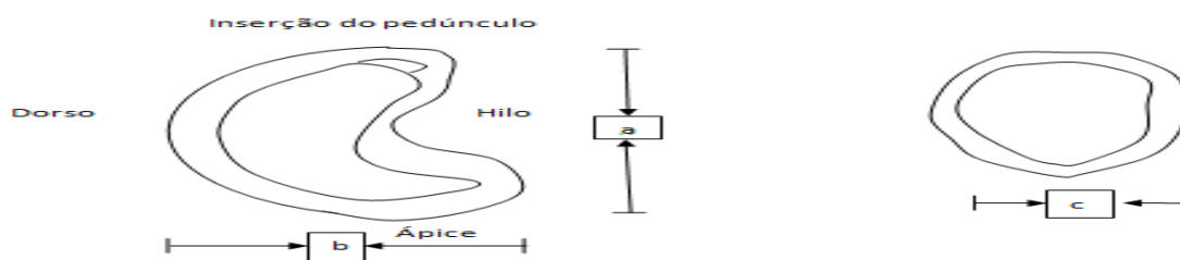
Figura 1. Dimensões características da castanha de caju. Comprimento (a), largura (b) e espessura (c), segundo Araújo; Ferraz, 2006.
