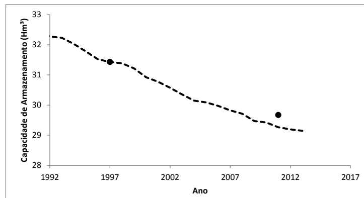
FIGURA 1. Simulação da redução da capacidade de armazenamento do reservatório Acarape do Meio para o período de 1991 a 2013.
