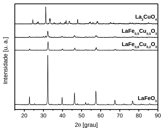
FIGURA 1. Difratogramas de raios X dos óxidos \text{LaFeO}_3 , \text{LaFe}_{0,8}\text{Cu}_{0,2}\text{O}_3 , \text{LaFe}_{0,5}\text{Cu}_{0,5}\text{O}_3 e \text{La}_2\text{CuO}_4 preparados por método convencional (citrato).
