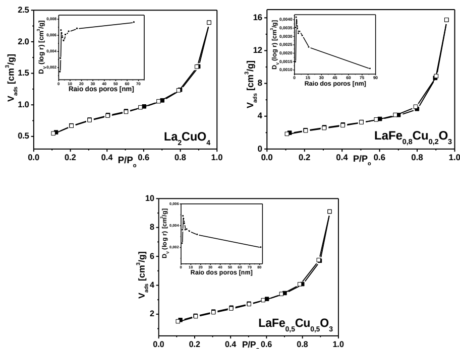
FIGURA 2. Isotermas de adsorção/dessorção de N 2 e distribuição BJH de tamanho de poros dos óxidos LaFe 1-x Cu x O 3 (x = 0; 0,2; 0,5) preparados pelo método citrato.
