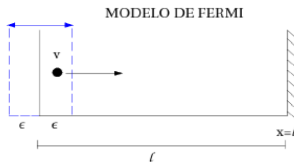
Figura 1: Esquema ilustrativo do modelo Fermi-Ulam
