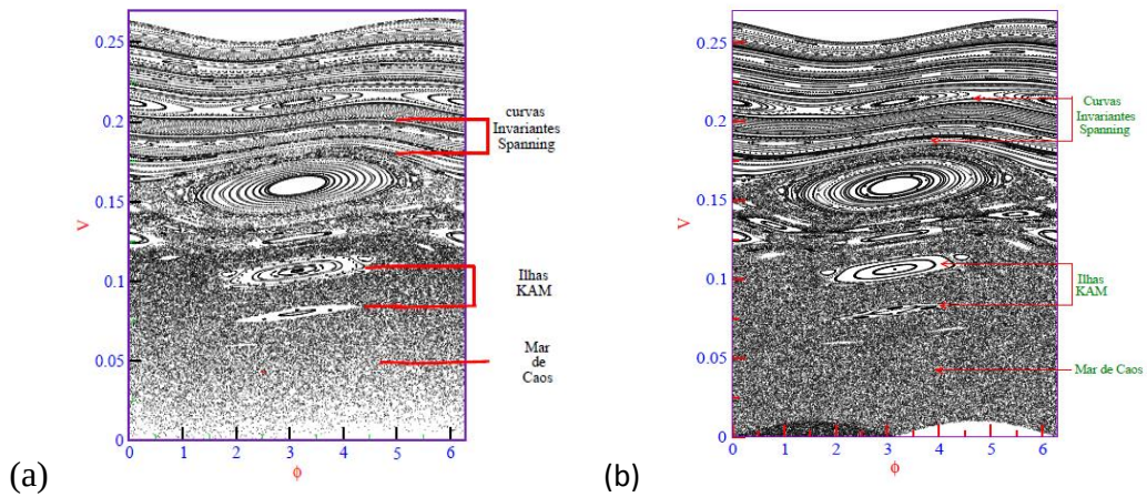
Figura 2: Espaço de fases do tipo misto para o modelo completo (a) e simplificado (b) do Acelerador de Fermi, onde o parâmetro de controle usado na construção das figuras foi \epsilon = 5 \times 10^{-3} .
