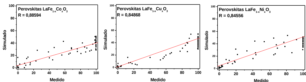
FIGURA 1. Dados medidos e simulados para os valores de teste de eficiência de conversão de NO com CO sobre os catalisadores \text{LaFe}_{1-x}\text{B}_x\text{O}_3 ( B = \text{Co}, \text{Cu}, \text{Ni} e x = 0; 0,2; 0,5 e 1).
